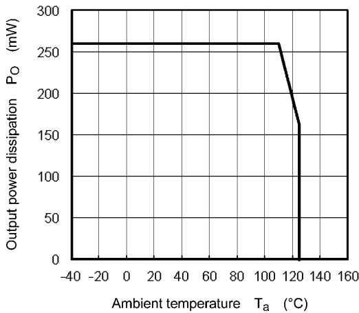
Fig. 12.2.3 P O - T a
