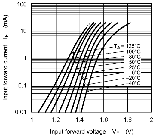
Fig. 12.2.1 I F - V F
