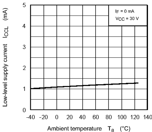
Fig. 12.2.5 I CCL - T a
