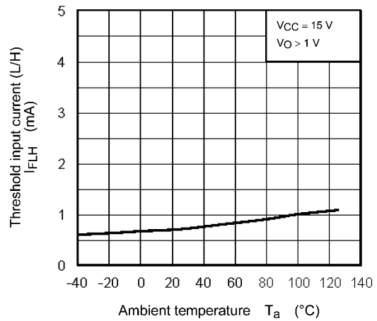
Fig. 12.2.4 I FLH - T a
