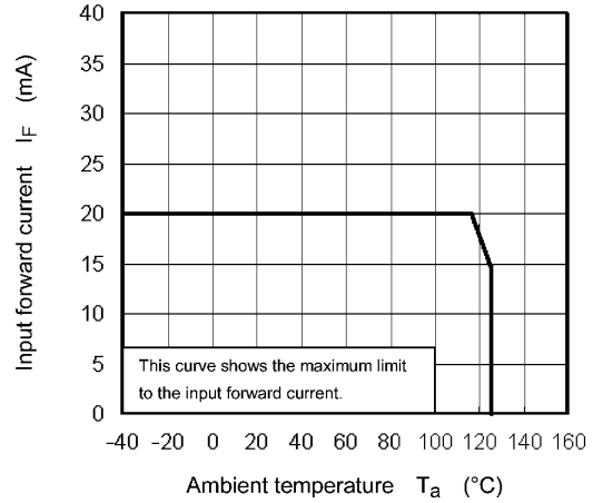
Fig. 12.2.2 I F - T a
