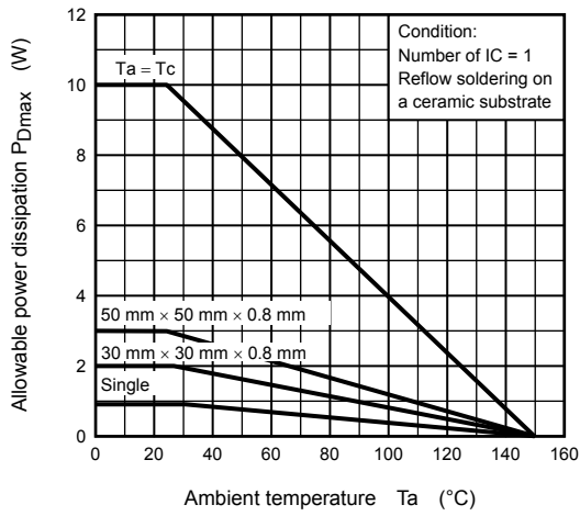
P_{Dmax} - T_a
