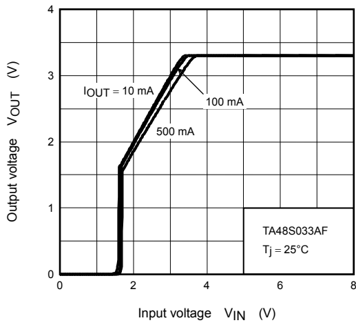
V_{OUT} - V_{IN}
