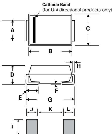
DO-214AB (SMC J-Bend)
