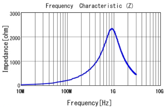
■ LQW15CNR33K1Z |Z|
