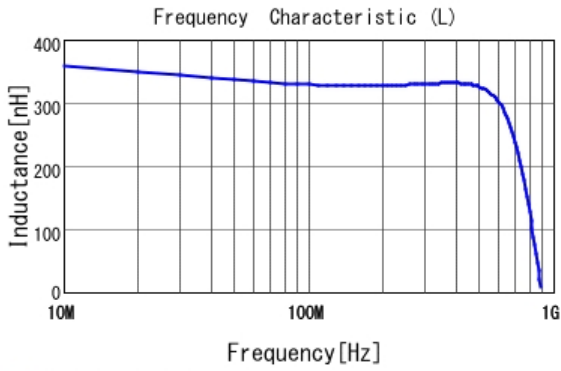
■ LQW15CNR33K1Z L
