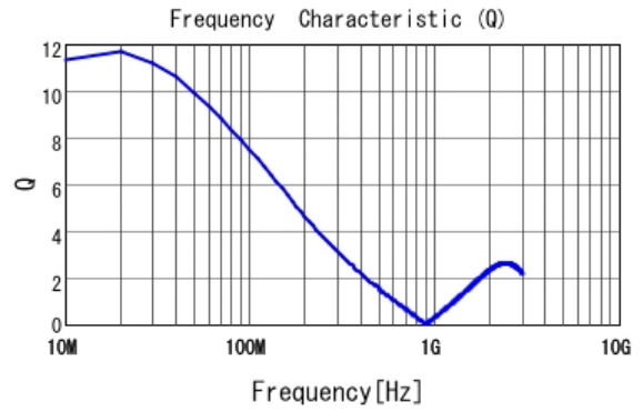
■ LQW15CNR33K1Z Q
