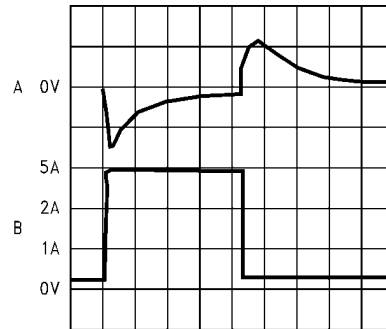
200 \mu sec/Div
