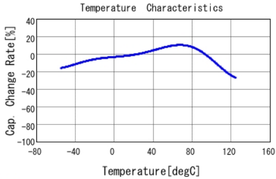
■ GRM32ED71A476ME15 C-Temp. capchange, DCO. 0V, ACO. 3Vrm
