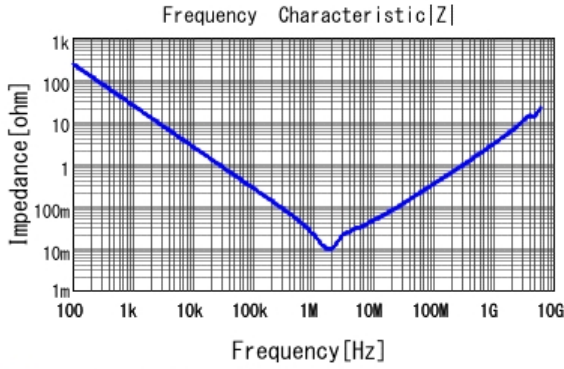
■ GCJ31CR71C106KA15 |Z| DCOV, 25degC
