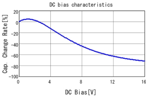
■ GCJ31CR71C106KA15 C-DC bias capchange, 25.0degC, AC1.
