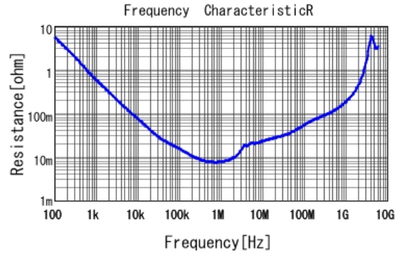
■ GCJ31CR71C106KA15 R DCOV, 25degC
