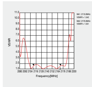
VSWR (INPUT)
