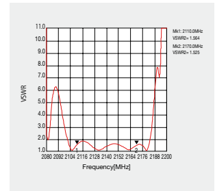
VSWR (OUTPUT)
