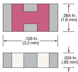
Case 18-2 (EIA 1206 / 3216)
