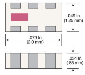
Case 15-1 (EIA 0805 / 2012)
