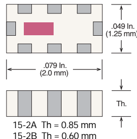
Case 15-2 (EIA 0805 / 2012)
