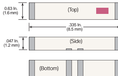
Case 46-1
