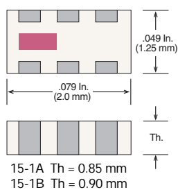
Case 15-1 (EIA 0805 / 2012)
