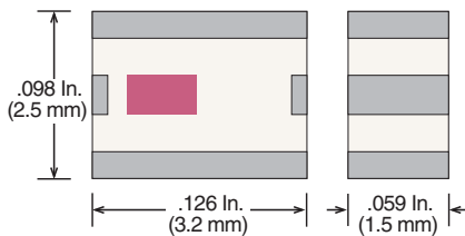
Case 41-1 (EIA 1210 / 3225)
