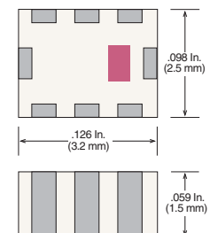
Case 41-2 (EIA 1210 / 3225)
