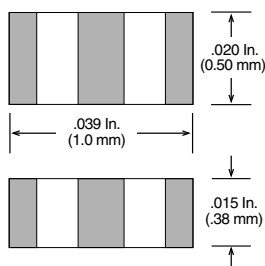
Case 07-1 (EIA 0402/ 1005)
