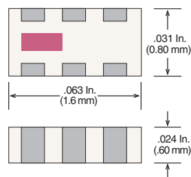
Case 14-1 (EIA 0603/ 1608)
